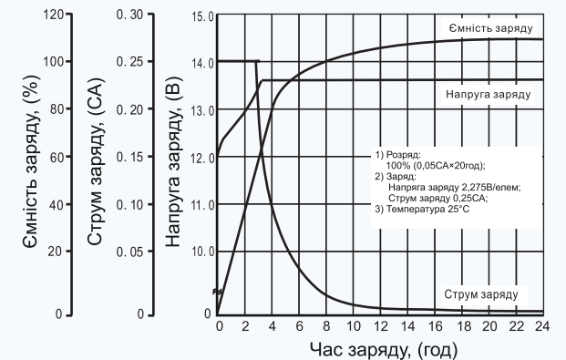
Криві заряду у буферному режимі
